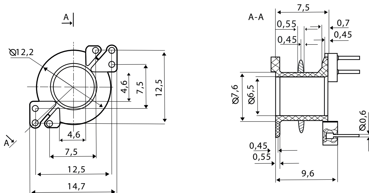
Габаритный чертеж
