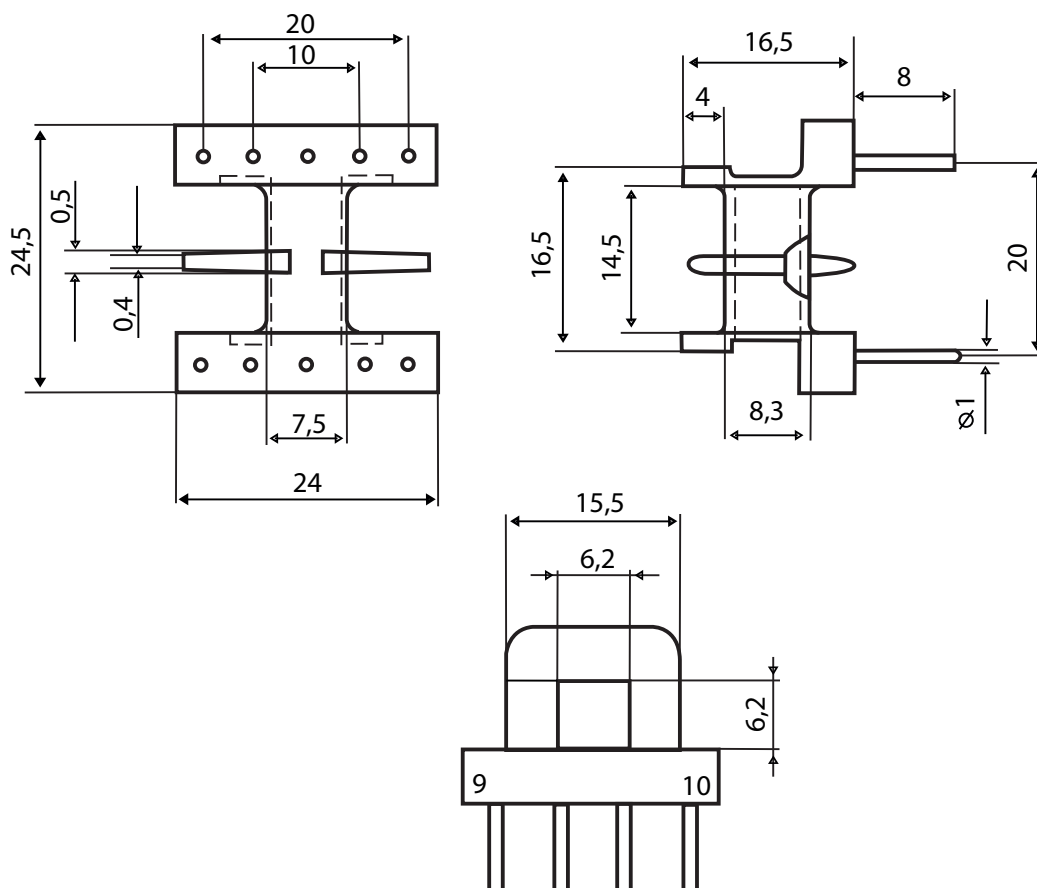
Габаритный чертеж
